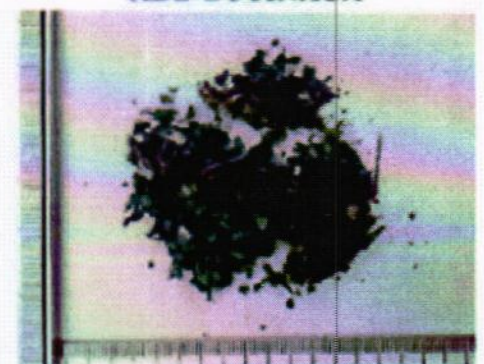
Mẫu thực vật khô cắt nhỏ chứa chất 4F-ABUTINACA
