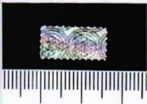
Mẫu tem giấy chứa chất 1cP-LSD
