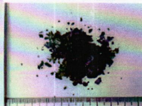
Mẫu thực vật khô cắt nhỏ chứa chất 4F-MDMB-BUTICA
